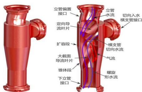
加强旋流器特殊单立管排水系统
