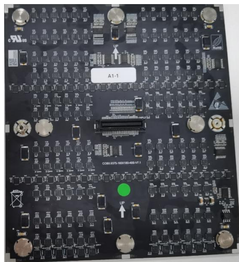
P0.9 单元模组
