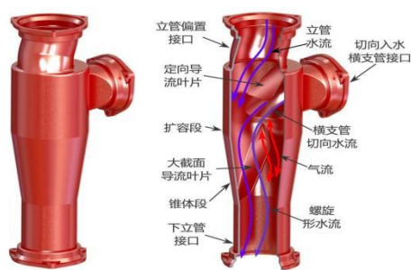
加强旋流器特殊单立管排水系统
