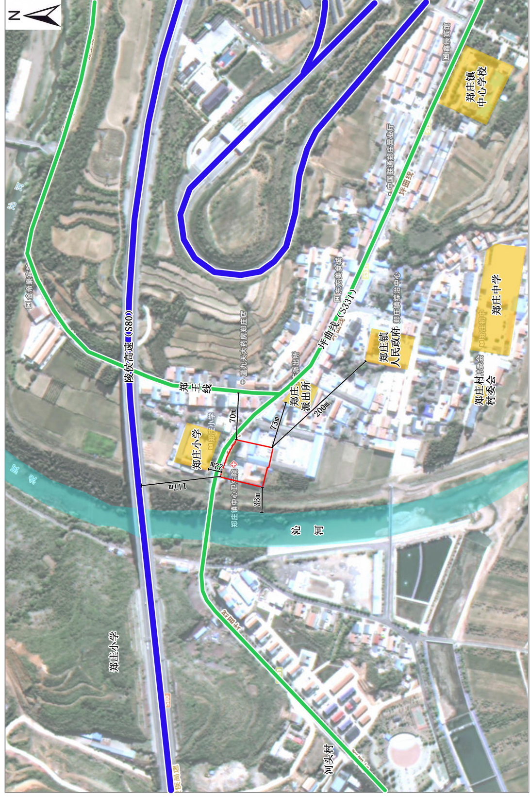
周边关系图
